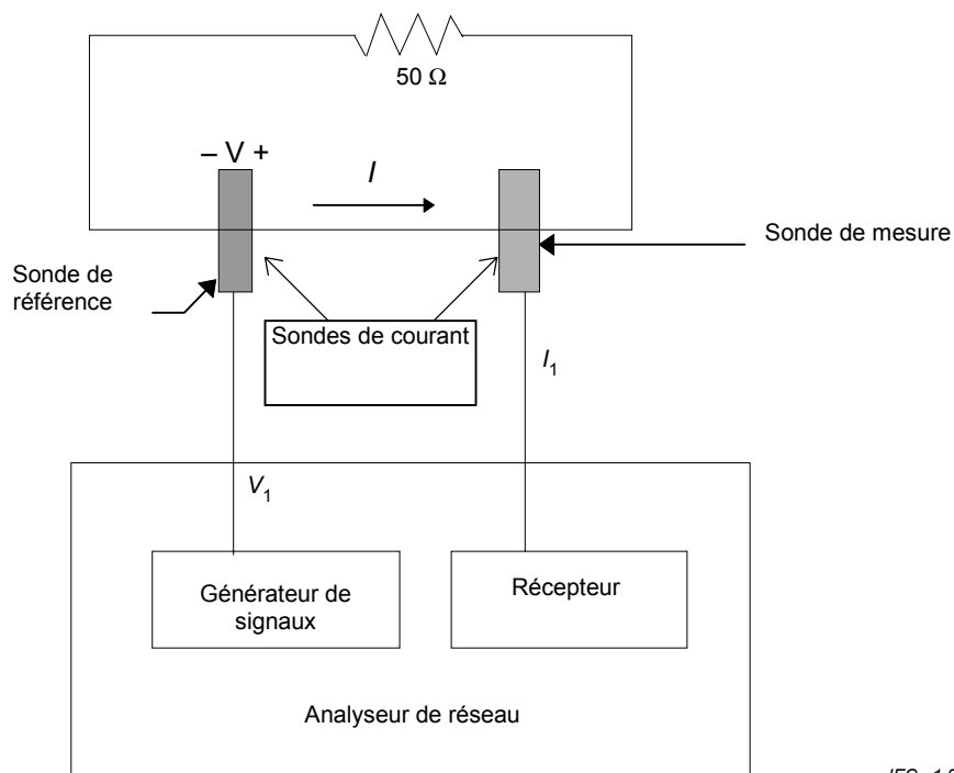
Figure C.5 – Dispositif d'étalonnage
