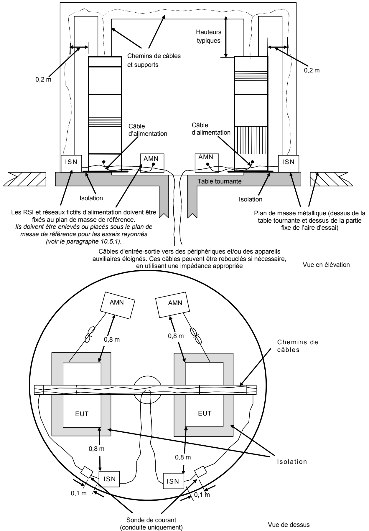
Figure 12 – Exemple de disposition d'essai pour appareils disposés à même le sol avec support vertical et câbles aériens (mesure d'émissions rayonnées et conduites)
