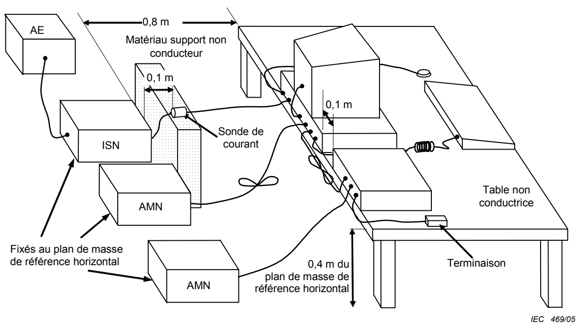
Figure 7 – Exemple de disposition d'essai pour appareils sur table (mesure d'émissions conduites – variante 2)
