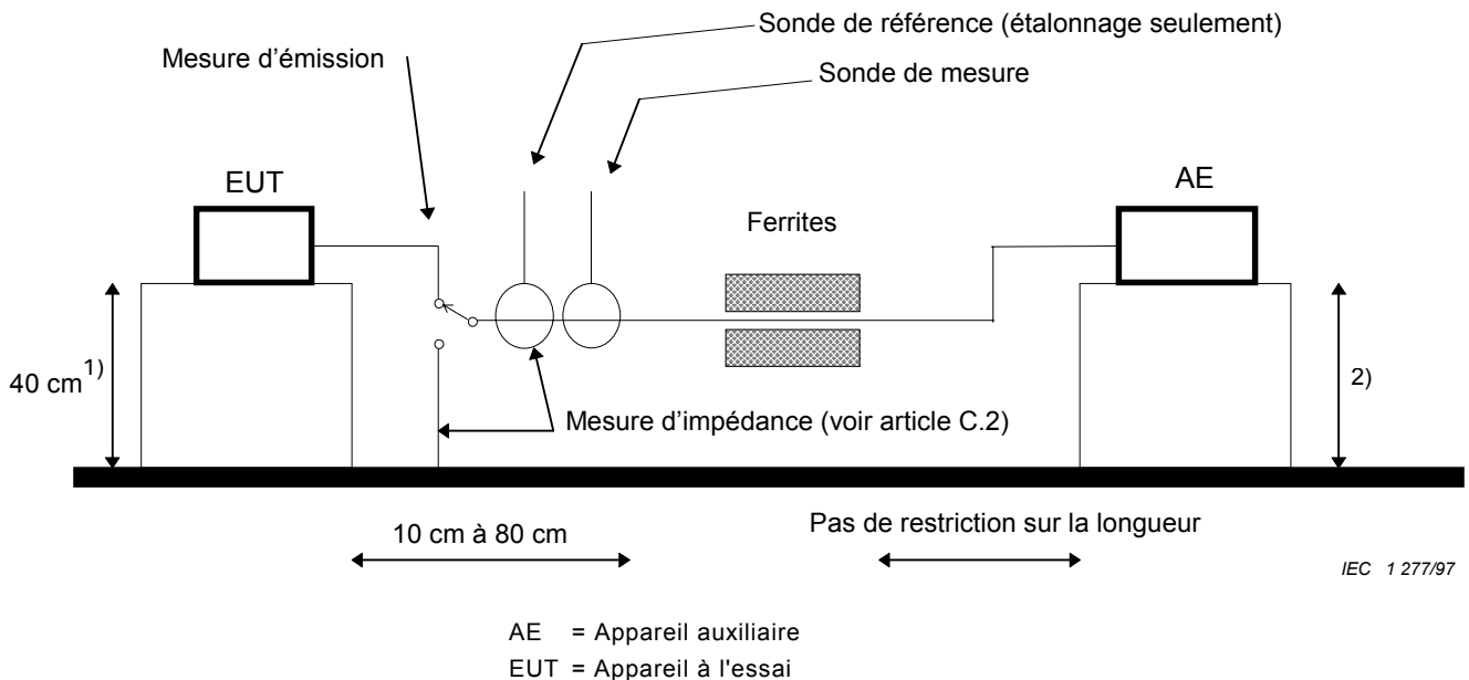
Figure C.4 – Utilisation d'aucune connexion au blindage et d'aucun RSI
